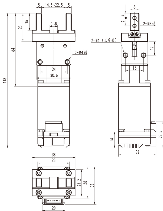
外形尺寸图
